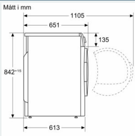
Måttskisser
